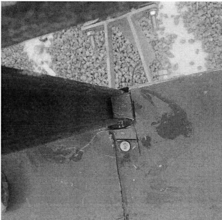
Instalación de pararrayos en cubierta cortando paneles y sin sellado.
