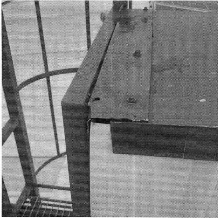
Instalación de escalera en cubierta cortando paneles y sin sellado.
